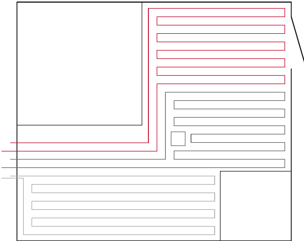
Beispiel 1: Raum mit 3 Heizkreisen parallel installiert
